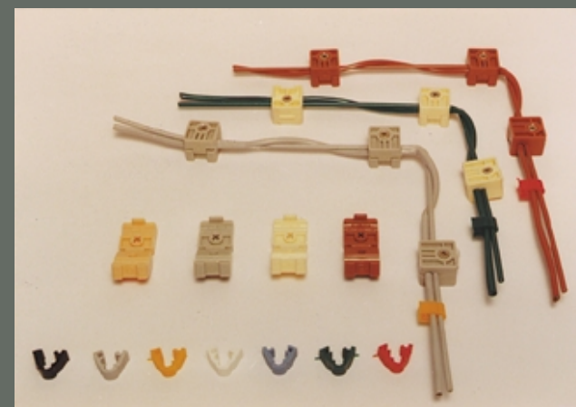
1990 カラープラスチック部品の長寿命化
