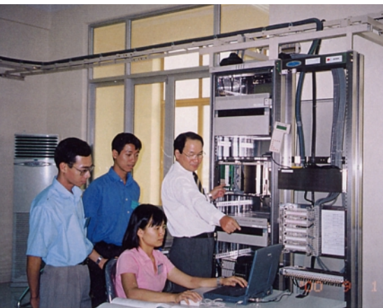
デジタル伝送の実習
