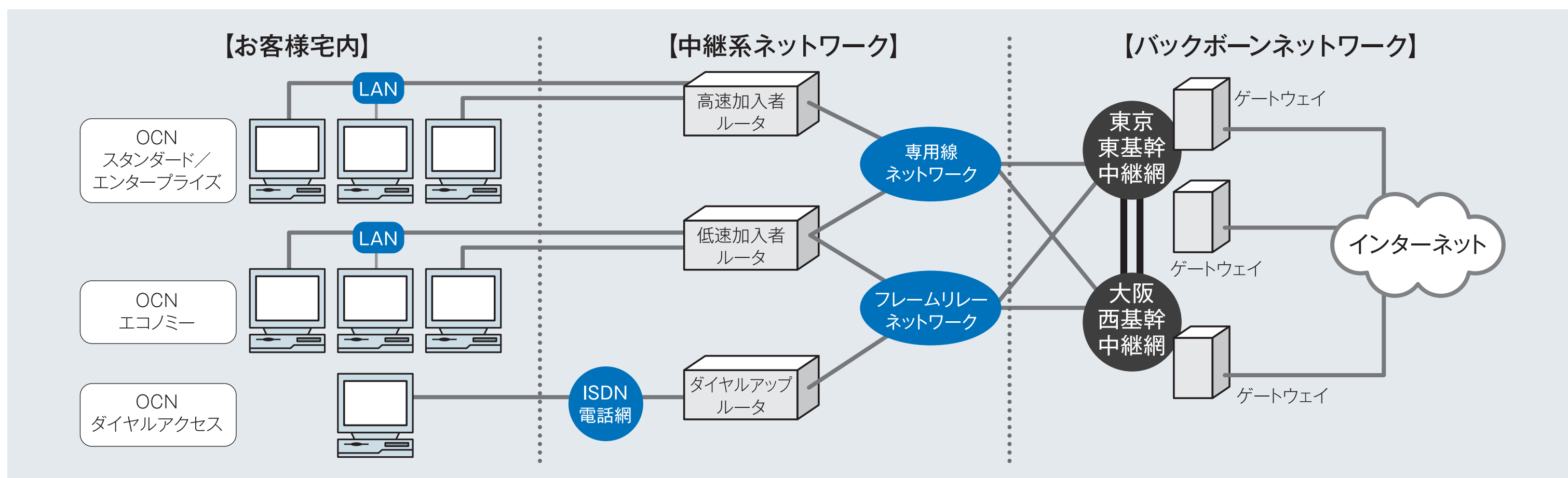
OCNのネットワーク概略図
