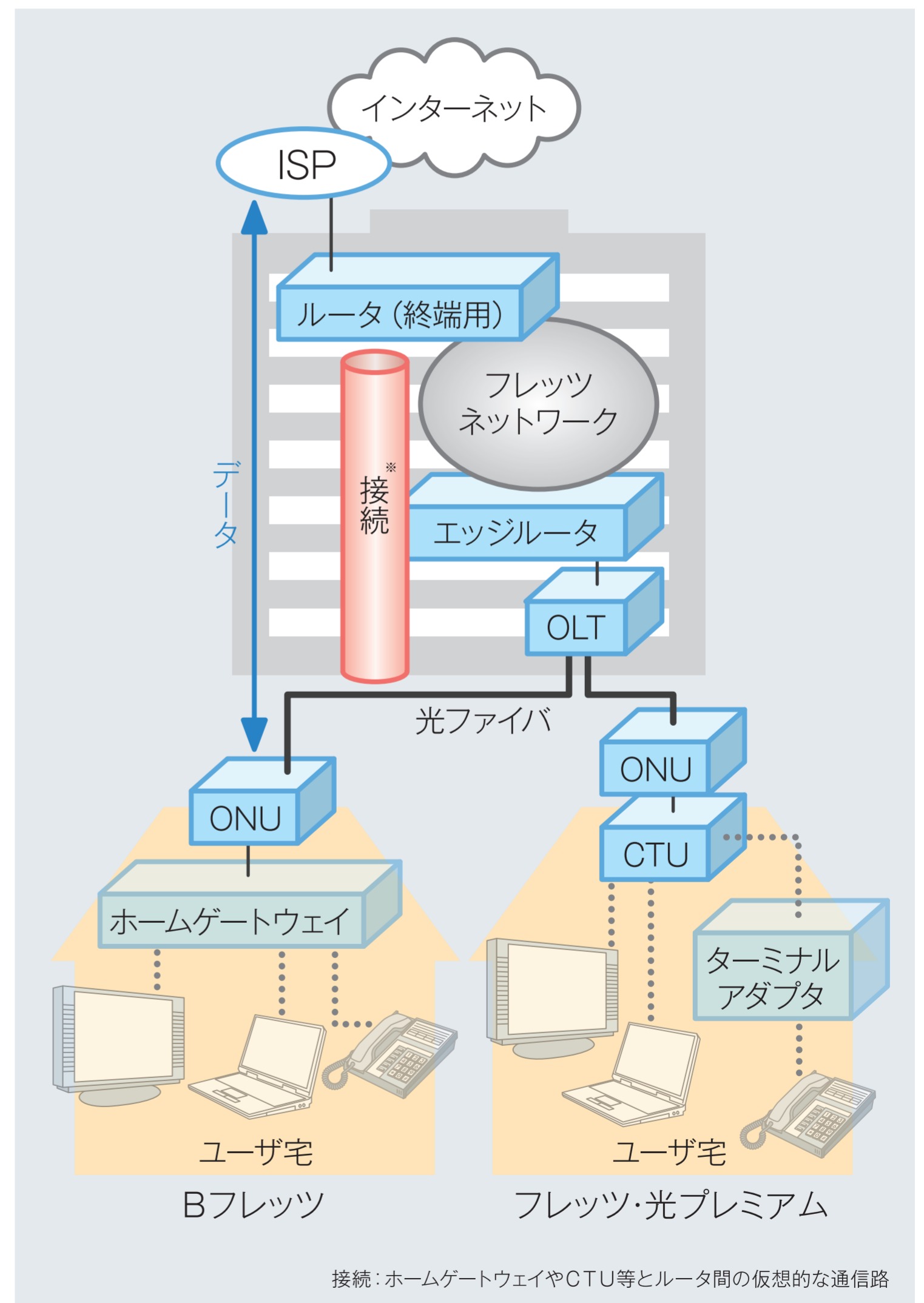
Bフレッツ、フレッツ・光プレミアム接続の例
